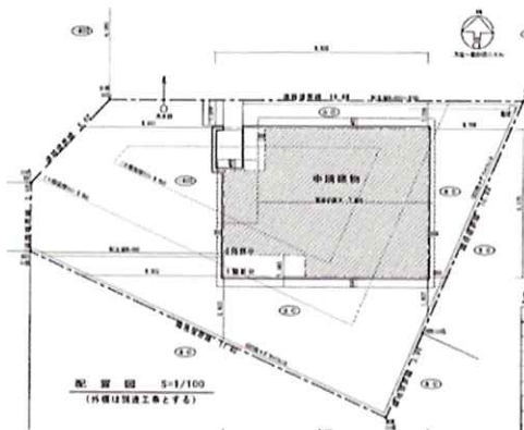
配置図
