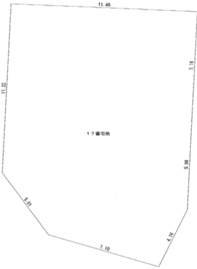
土地寸法図
